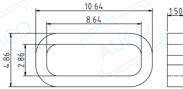
建议胶圈尺寸
