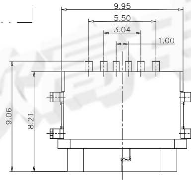
TYPE C 6P 沉板防水母座 (外壳4脚插板, 端子SMT)
