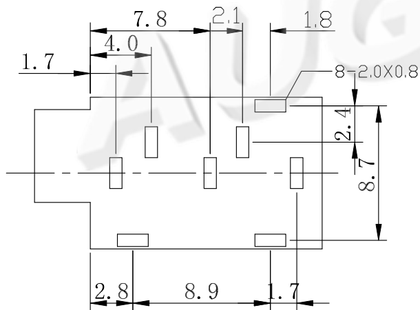
线路板安装结构示意图
