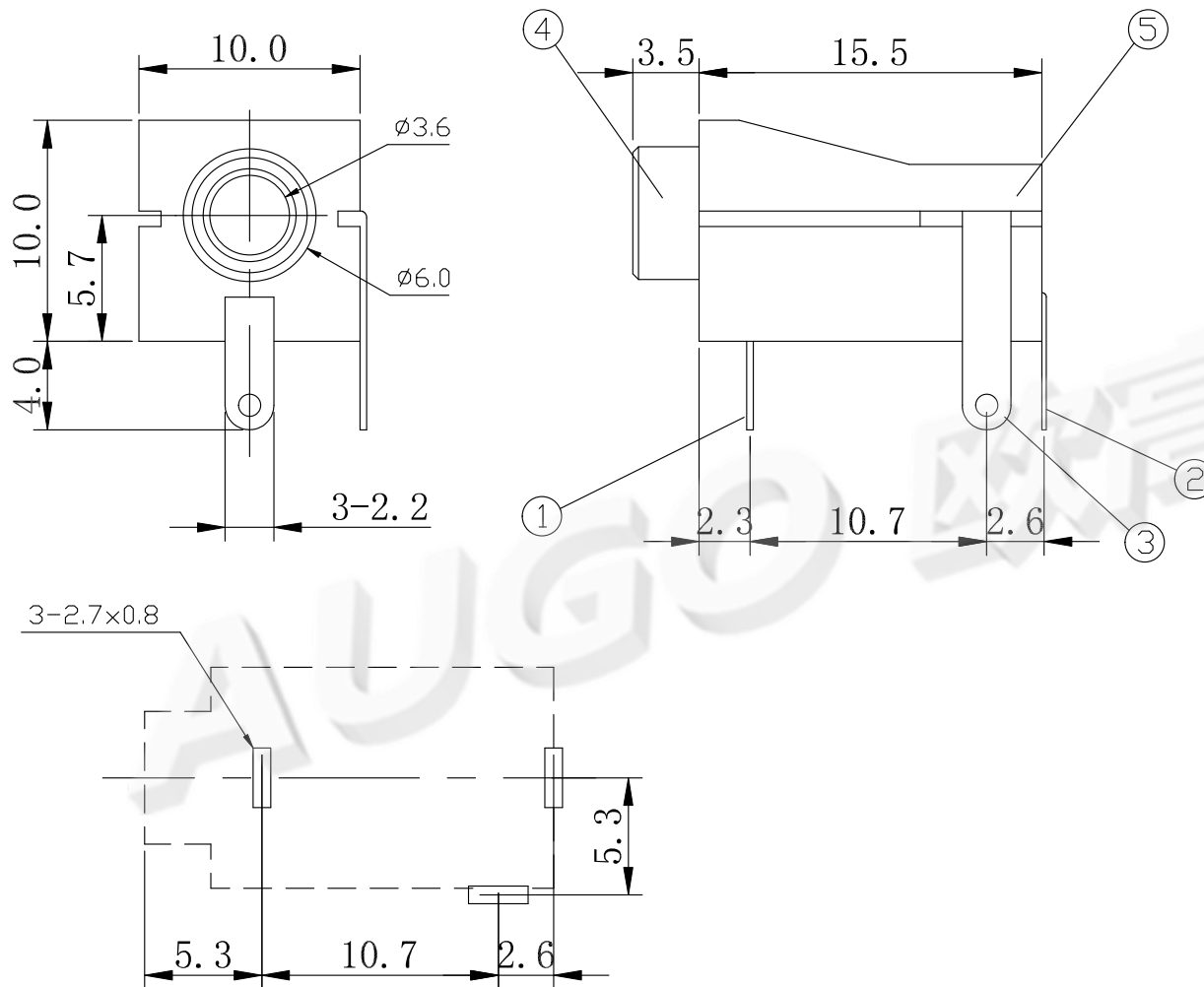
线路板安装尺寸示意图
