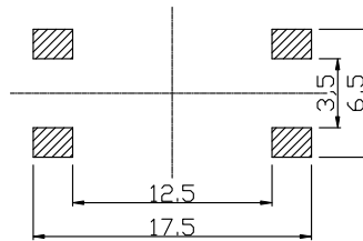
PCB. 焊接图
