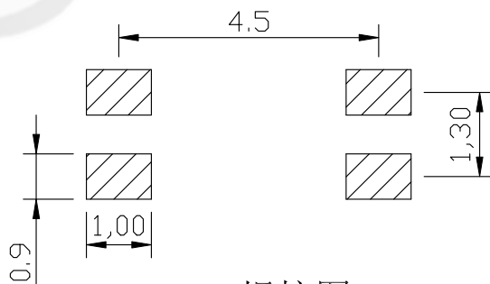
PCB. 焊接图
