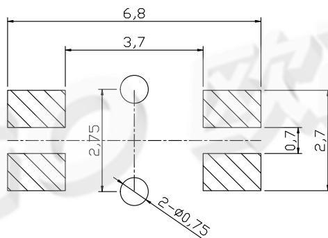
PCB. 焊接图
