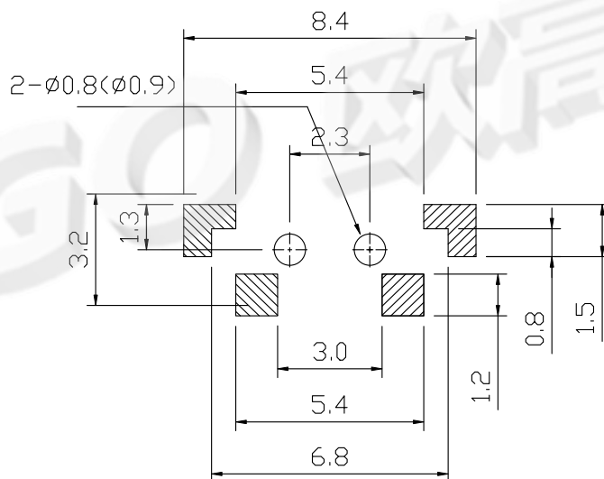
PCB. 焊接图
