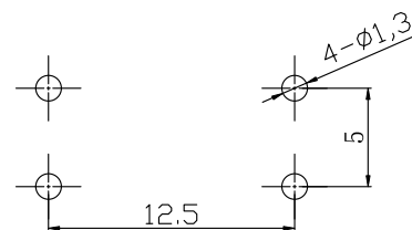
PCB. 焊接图
