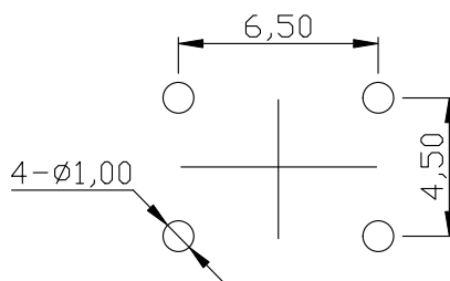
PCB. 焊接图
