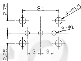
PCB. 焊接图
