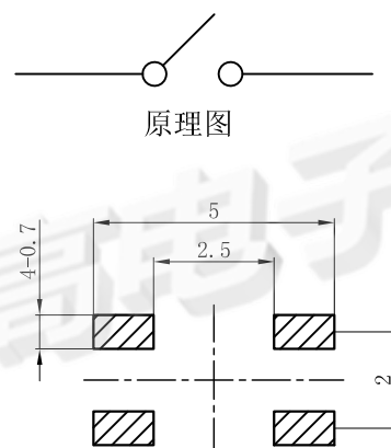
安装参考图
