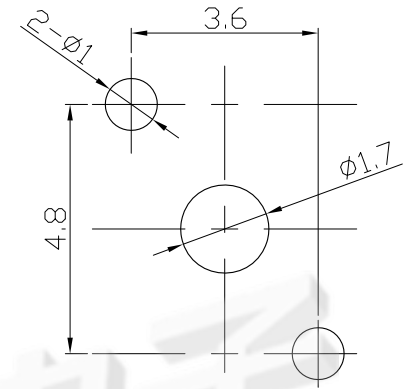
安装尺寸图
